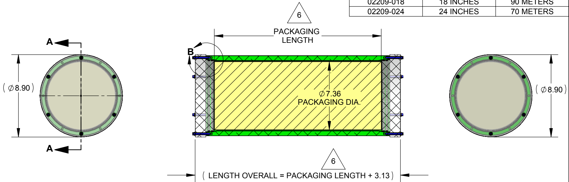
SECTION A-A SCALE 1 : 6
