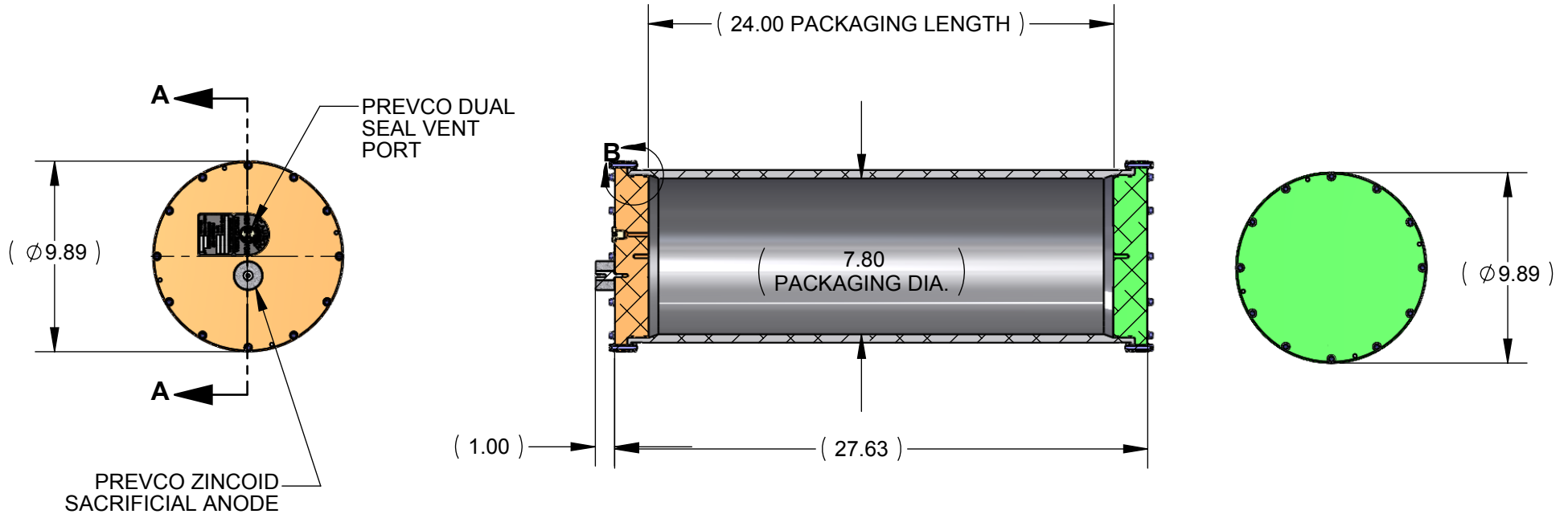
SECTION A-A
